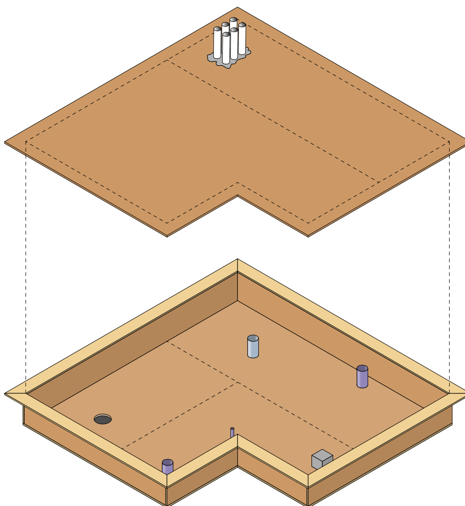
Figur 2. Prøvestand til måling af lufttæthed af materialer anvendt til radonsikring. Samlinger i membranen er vist med stiplede linjer. Prøvestanden er vist med placeringen af hjørner og gennemføringer.
