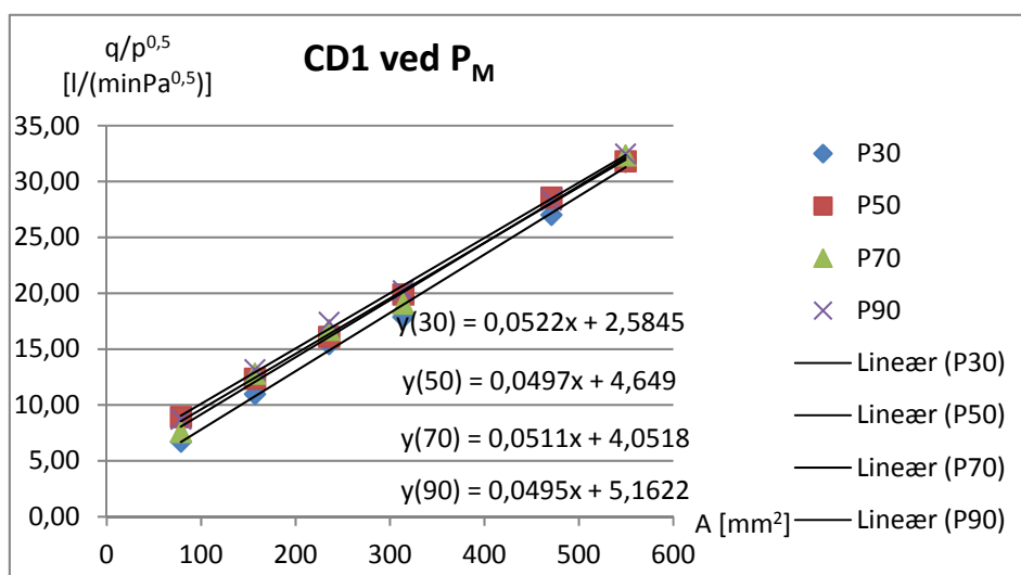
Figur 6 Prøvningsresultater: Relativ luftstrøm ved forskellige tryk q/p^{0,5} for forskellige blændeåbninger A etableret i membranens overside.
